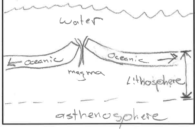
Divergent (Ocean-Ocean)
